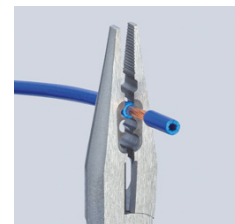
Удаление изоляции
